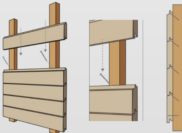
VOORBEELD MONTAGE GEVELBEKLEDING MES EN GROEF
